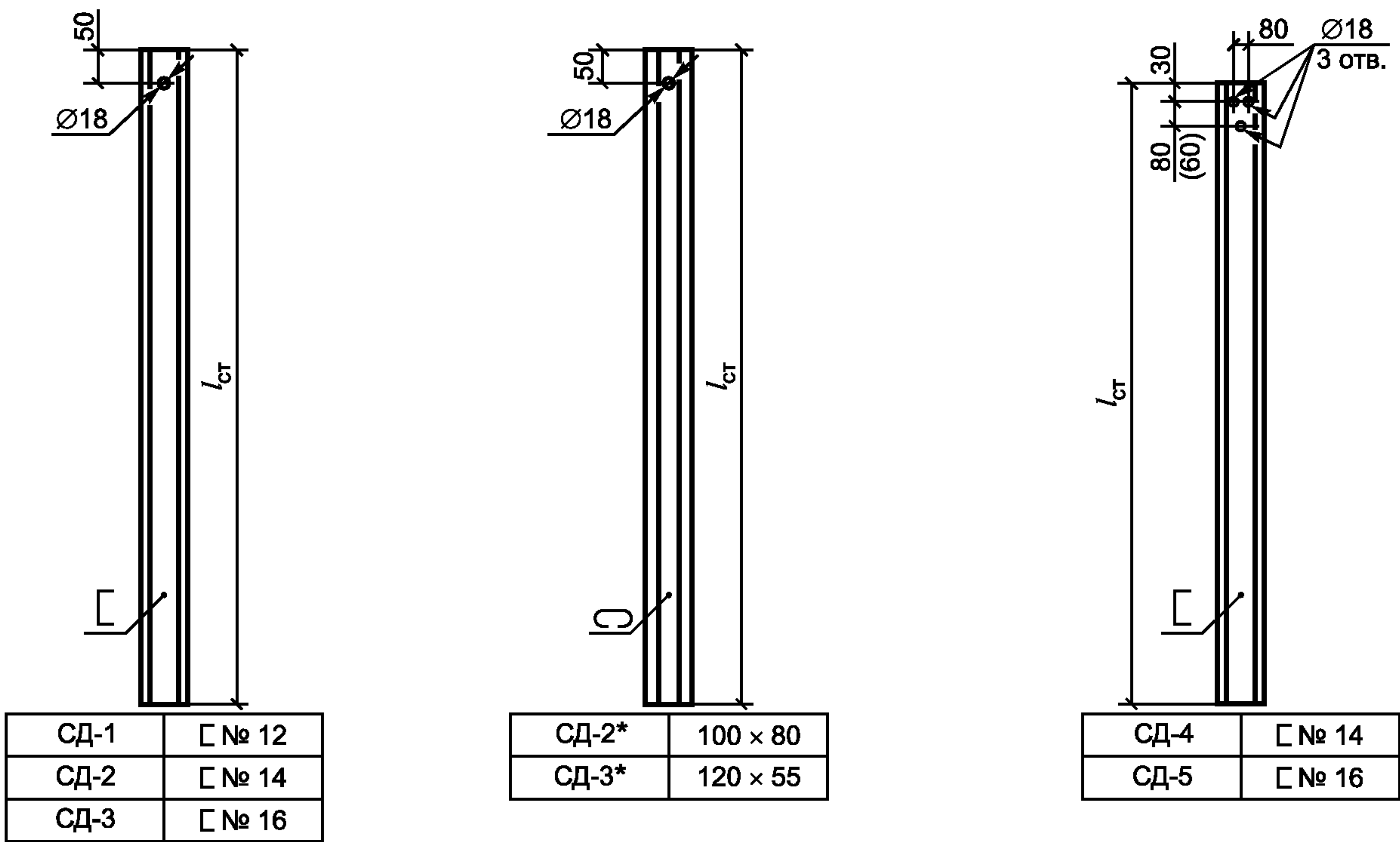
а) Для односторонних ограждений с жесткими консолями
