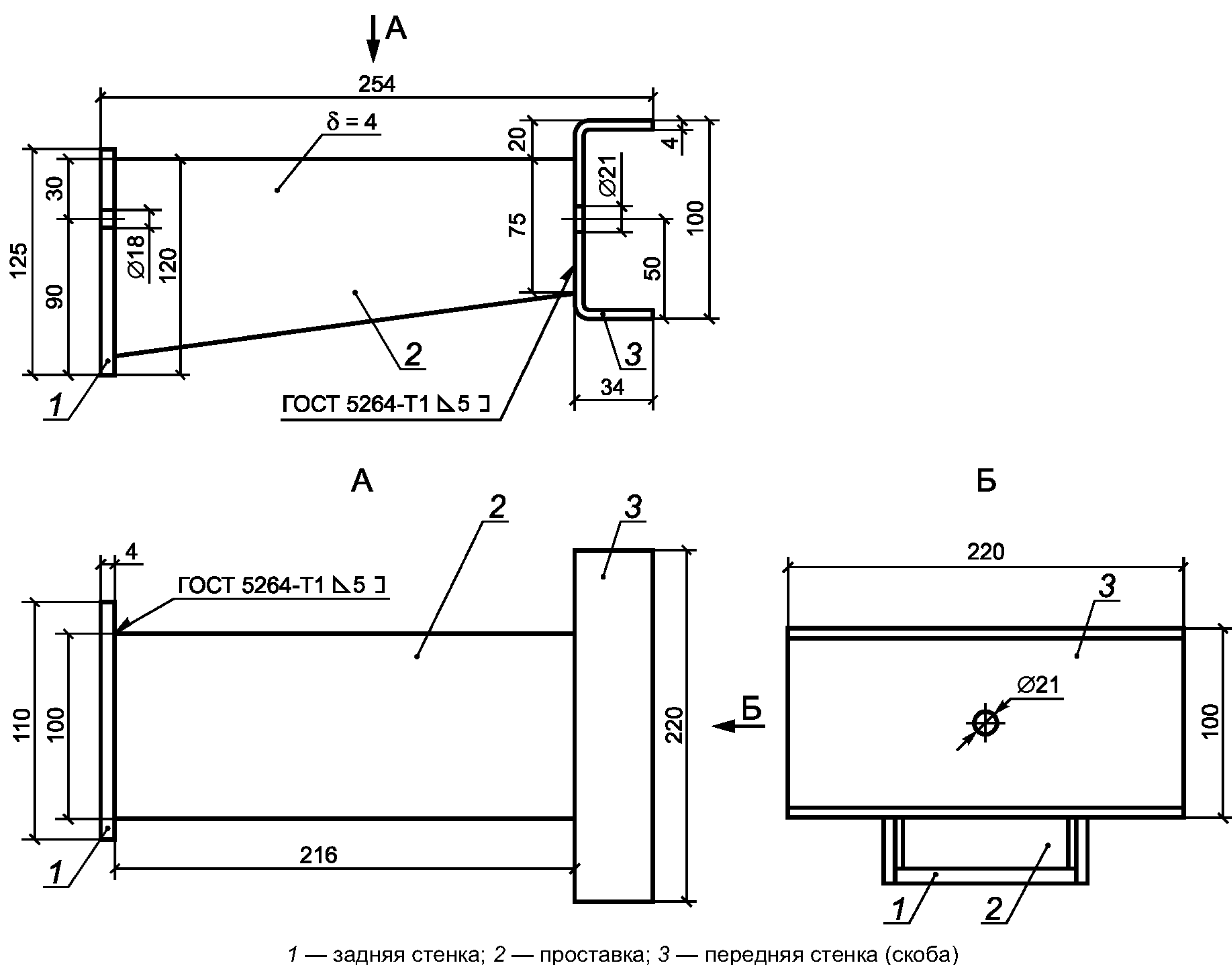
Рисунок 8 — Консоль жесткая КЖ
