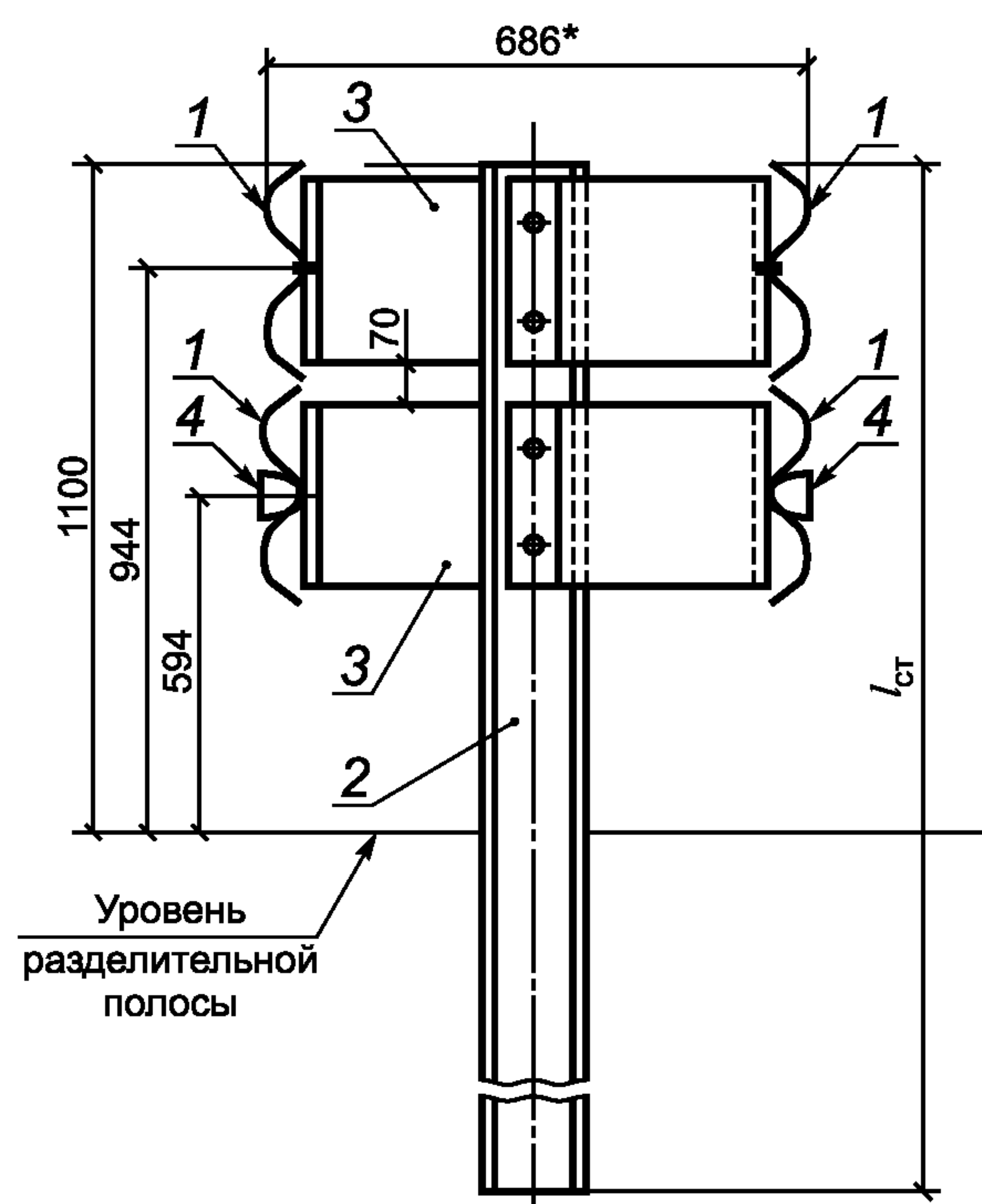
г) Двухстороннее двухъярусное ограждение
