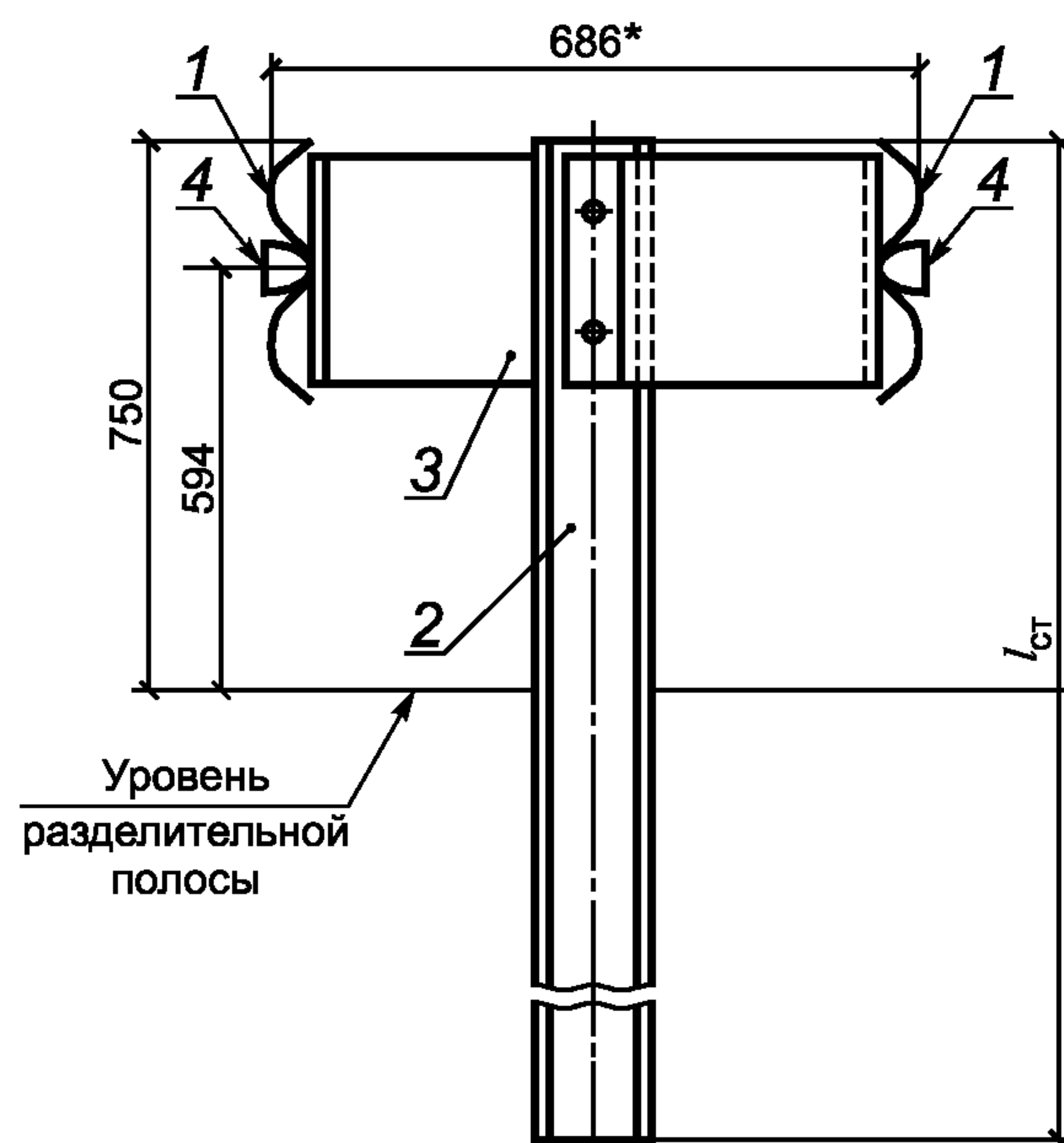
б) Двухстороннее одноярусное ограждение
