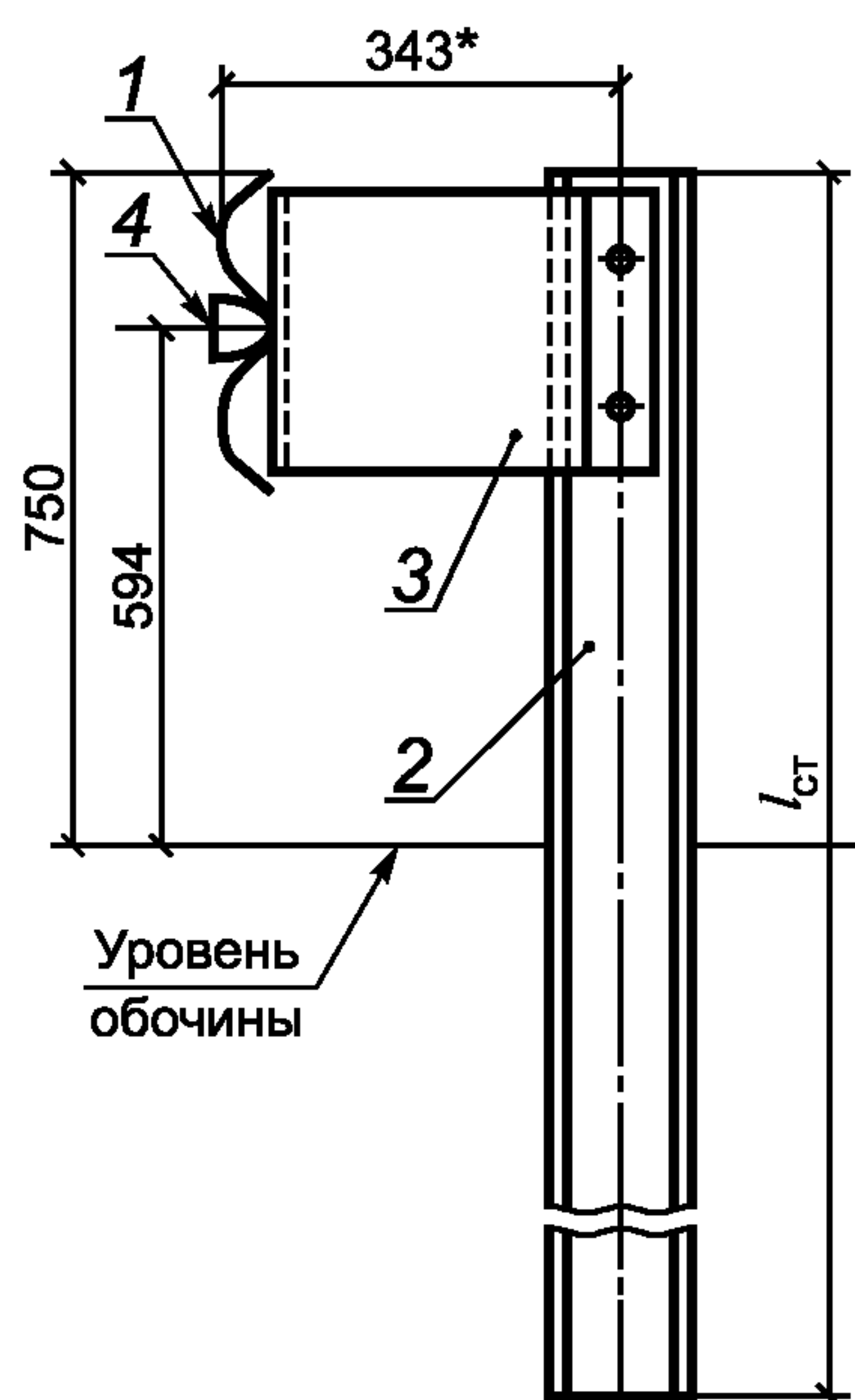
а) Одностороннее одноярусное ограждение
