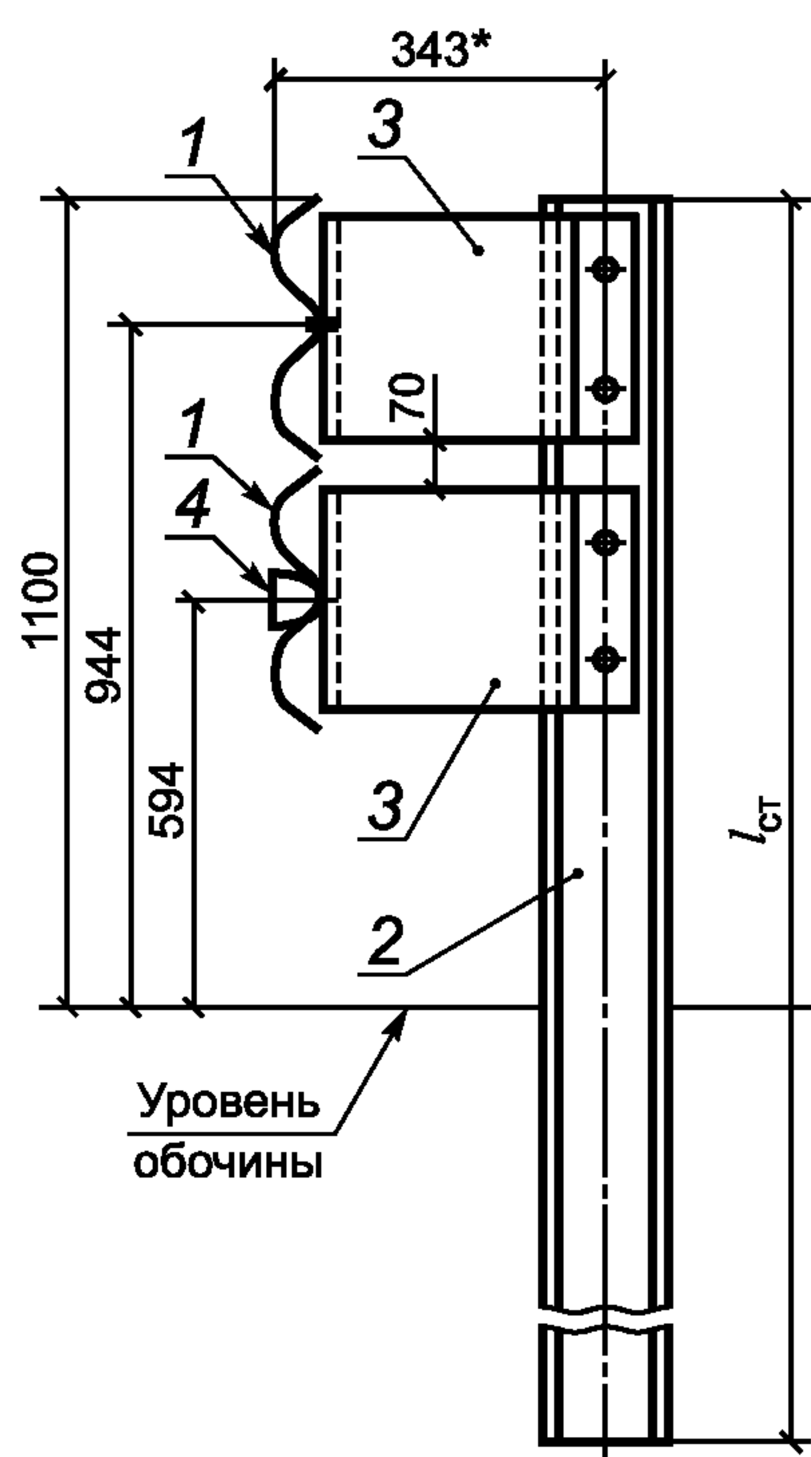
в) Одностороннее двухъярусное ограждение
