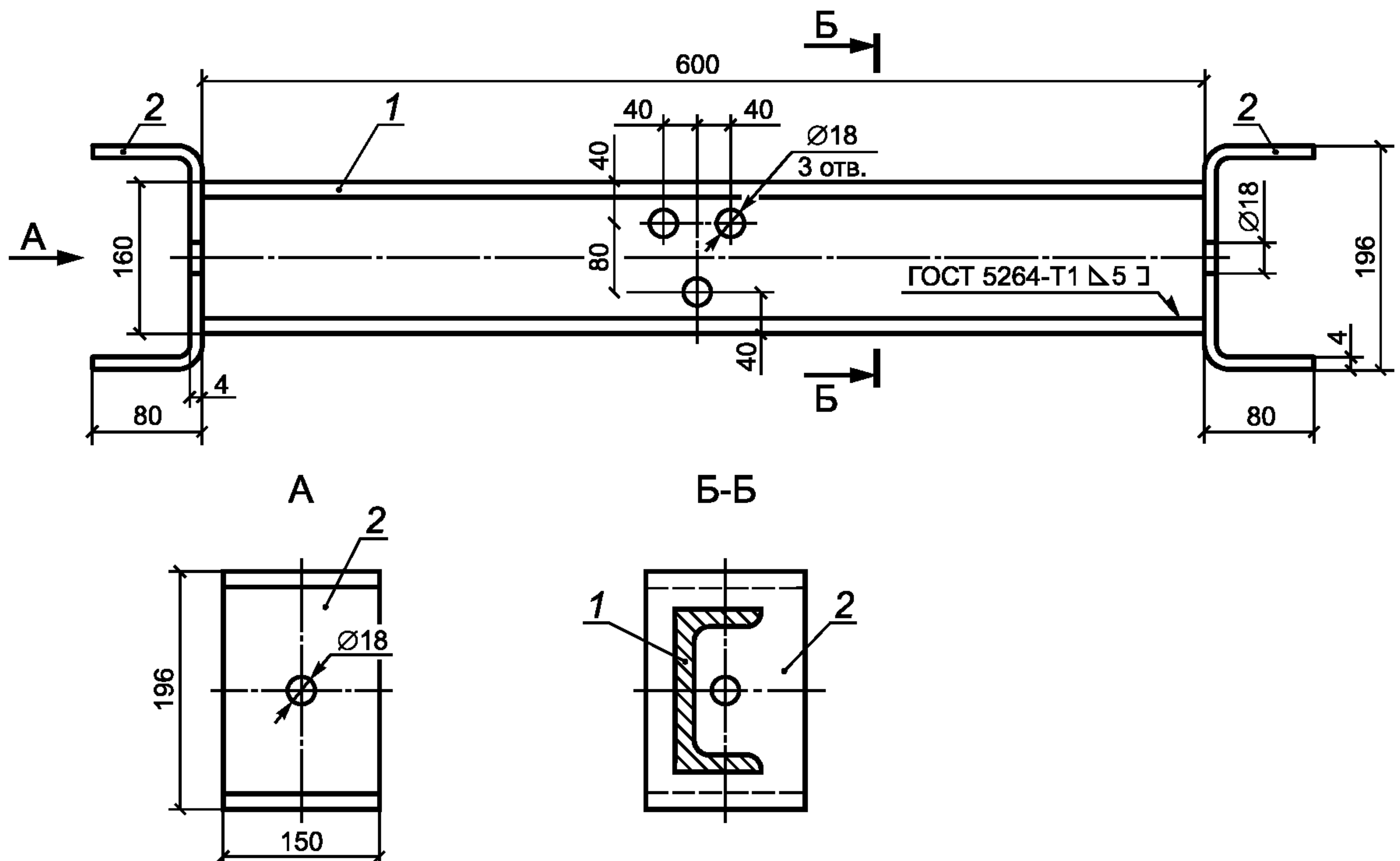
Рисунок 8 — Консоль жесткая КЖ
