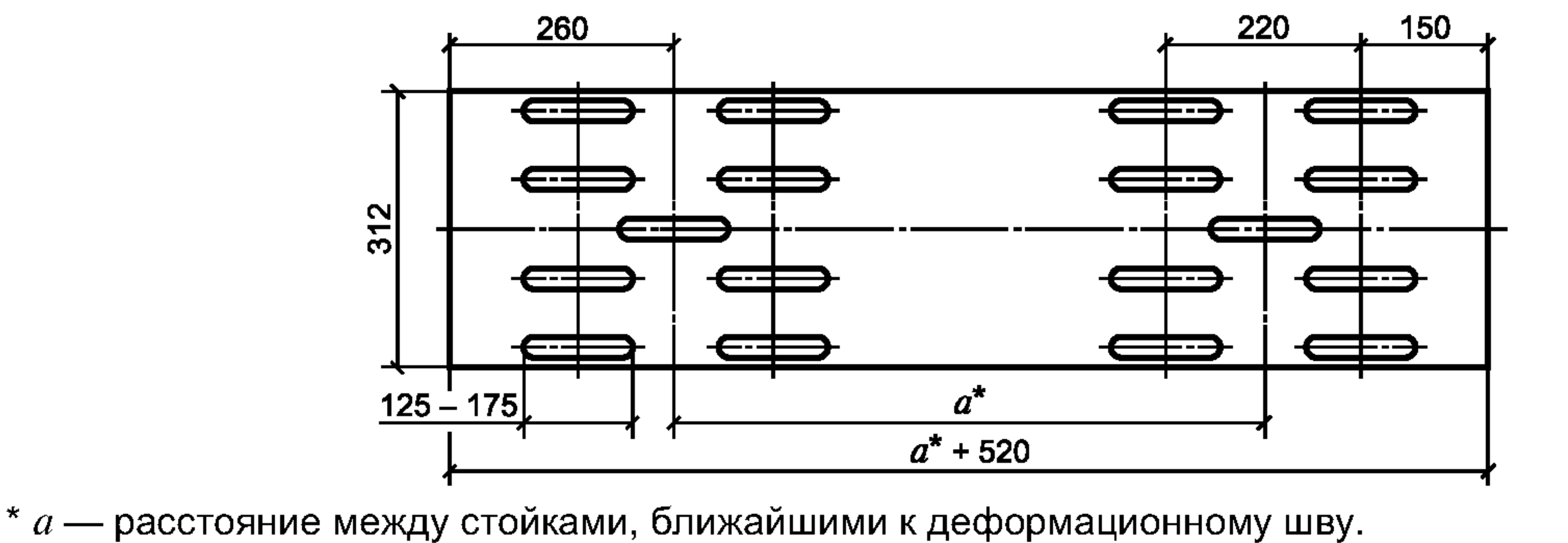
Рисунок 6 — Секция балки-вставки СБВ над деформационным швом
