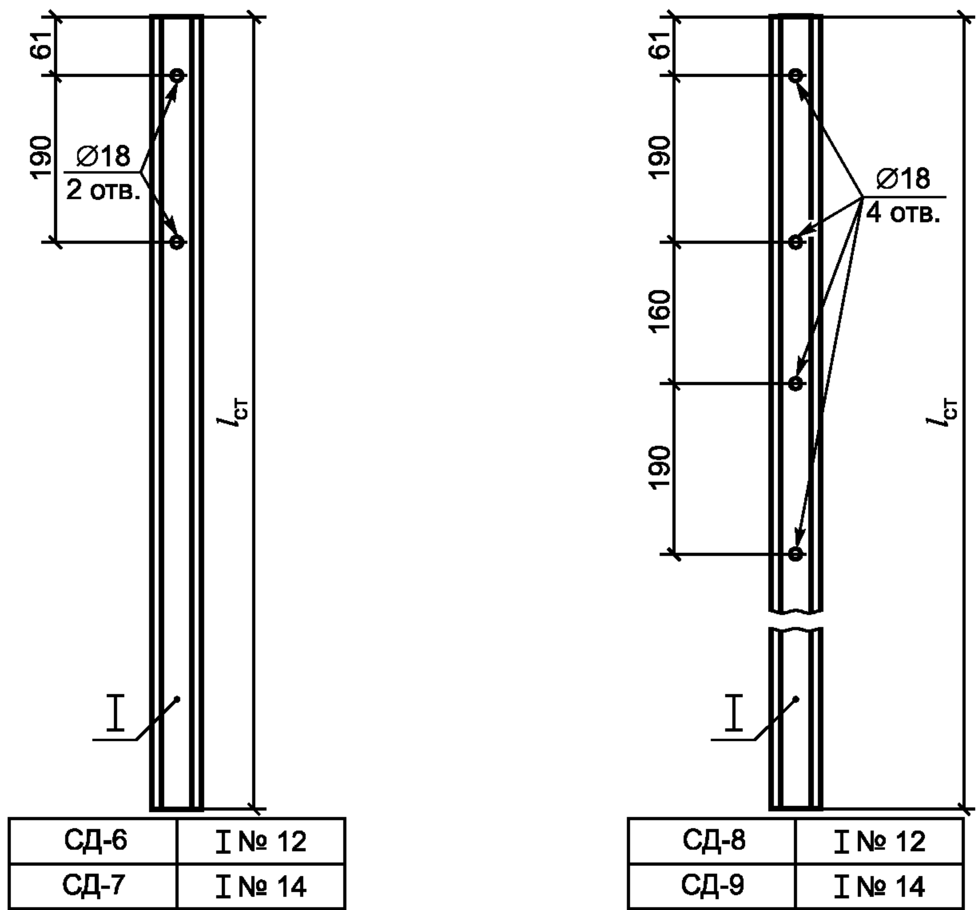
г) Для односторонних ограждений с консолью-амортизатором с одним ярусом балки
