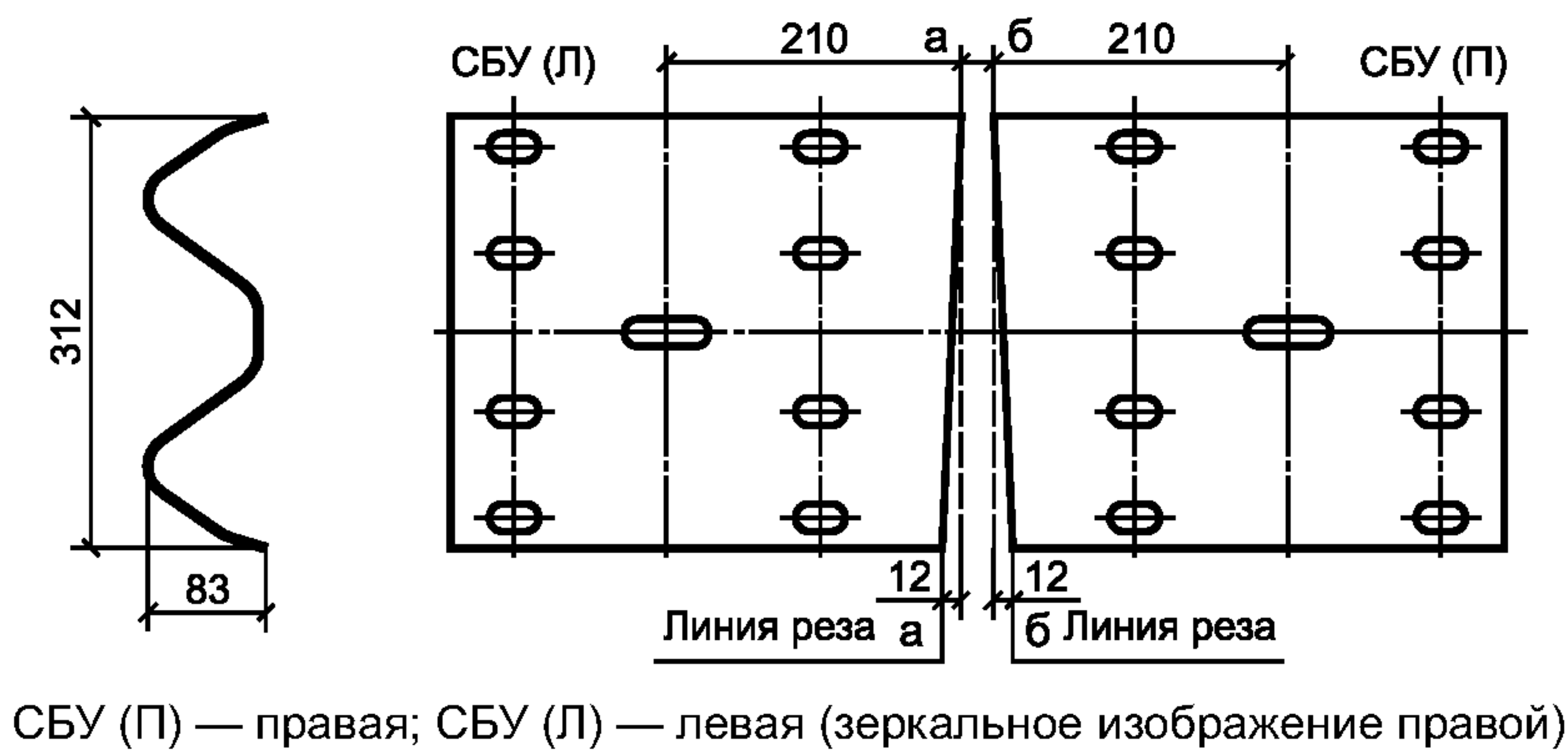
Рисунок 5 — Секция балки угловой СБУ
