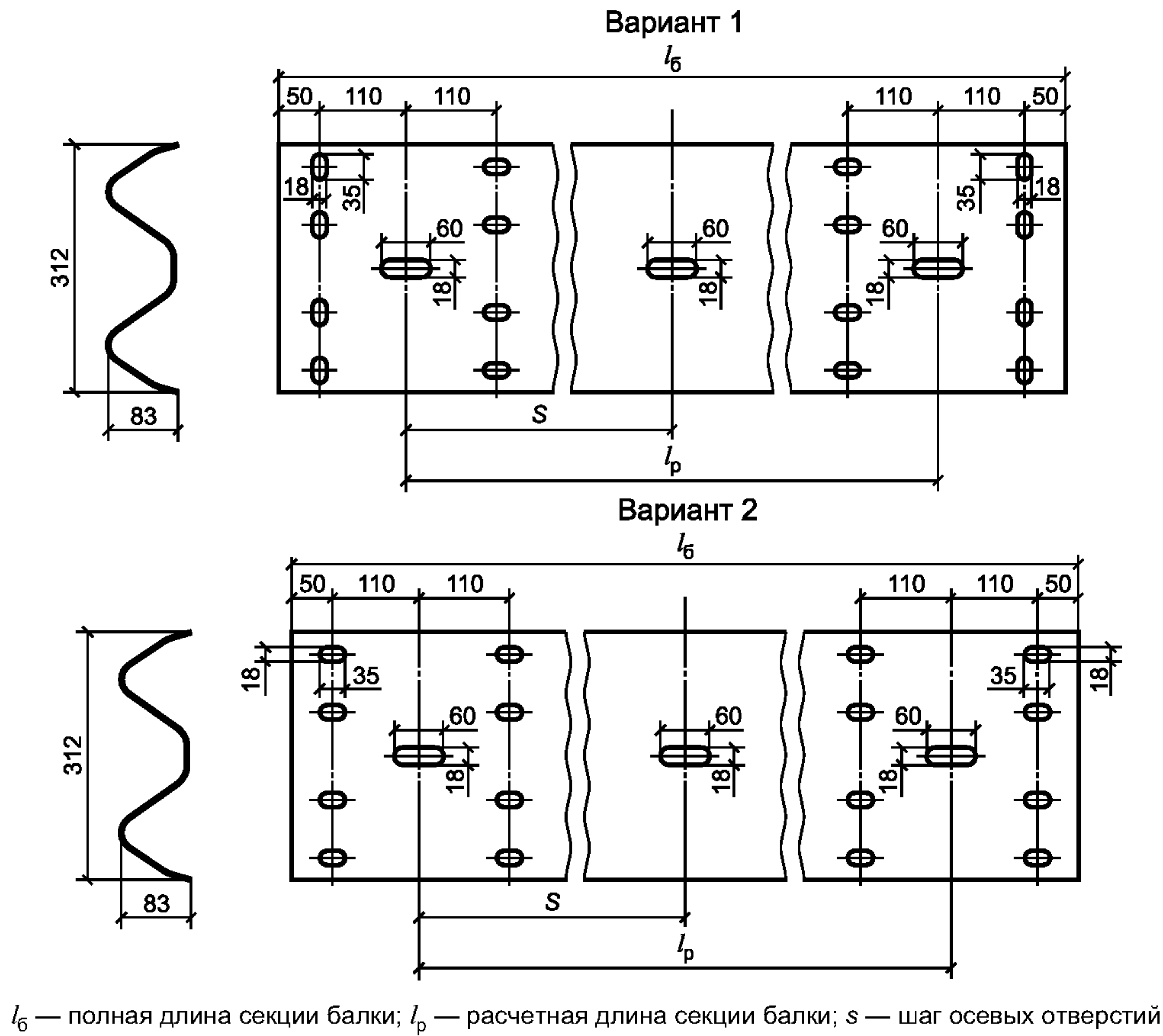
Рисунок 4 — Секция балки ограждений СБ
